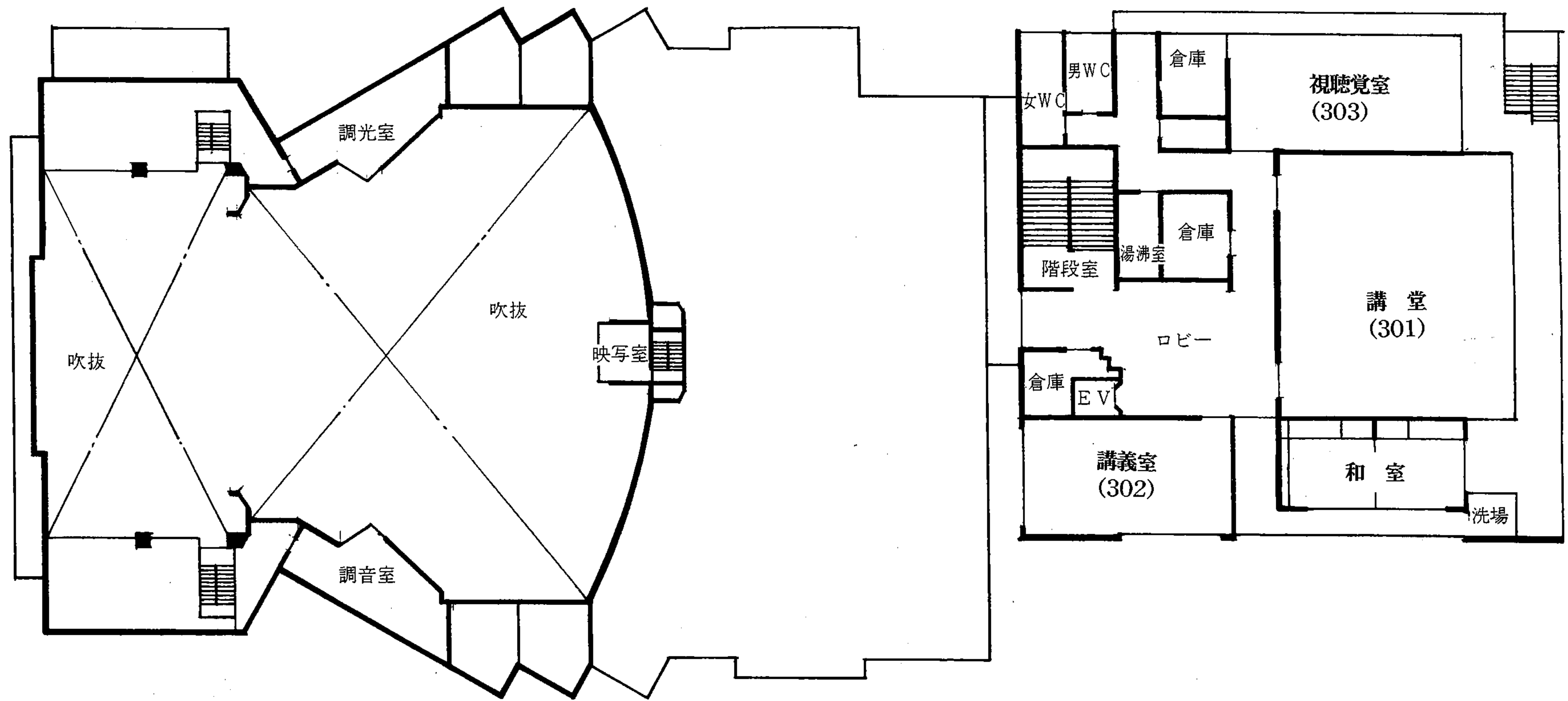
3 階平面
