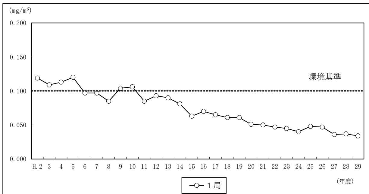
図 3－4 浮遊粒子状物質の経年変化（日平均値の2%除外値）
