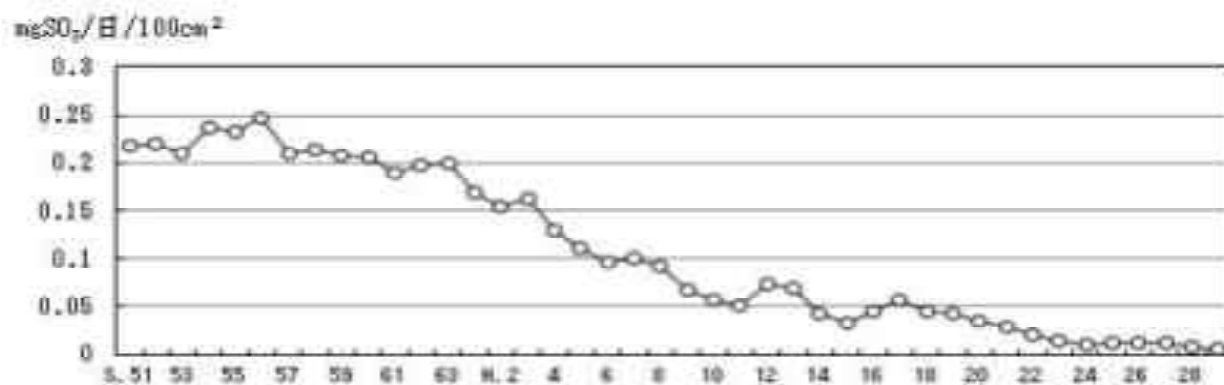
図3-8 硫黄酸化物年平均値経年変化
