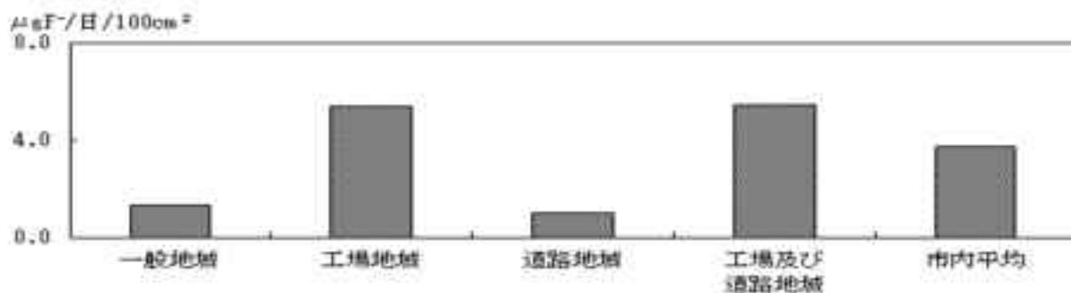
図3-13 平成29年度ふっ素イオン地域別年平均値
