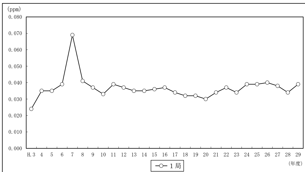
図 3-5 光化学オキシダントの年平均値経年変化
