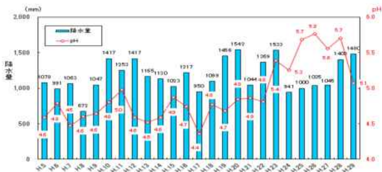
図3-26 降水量とpH年平均値の経年変化
