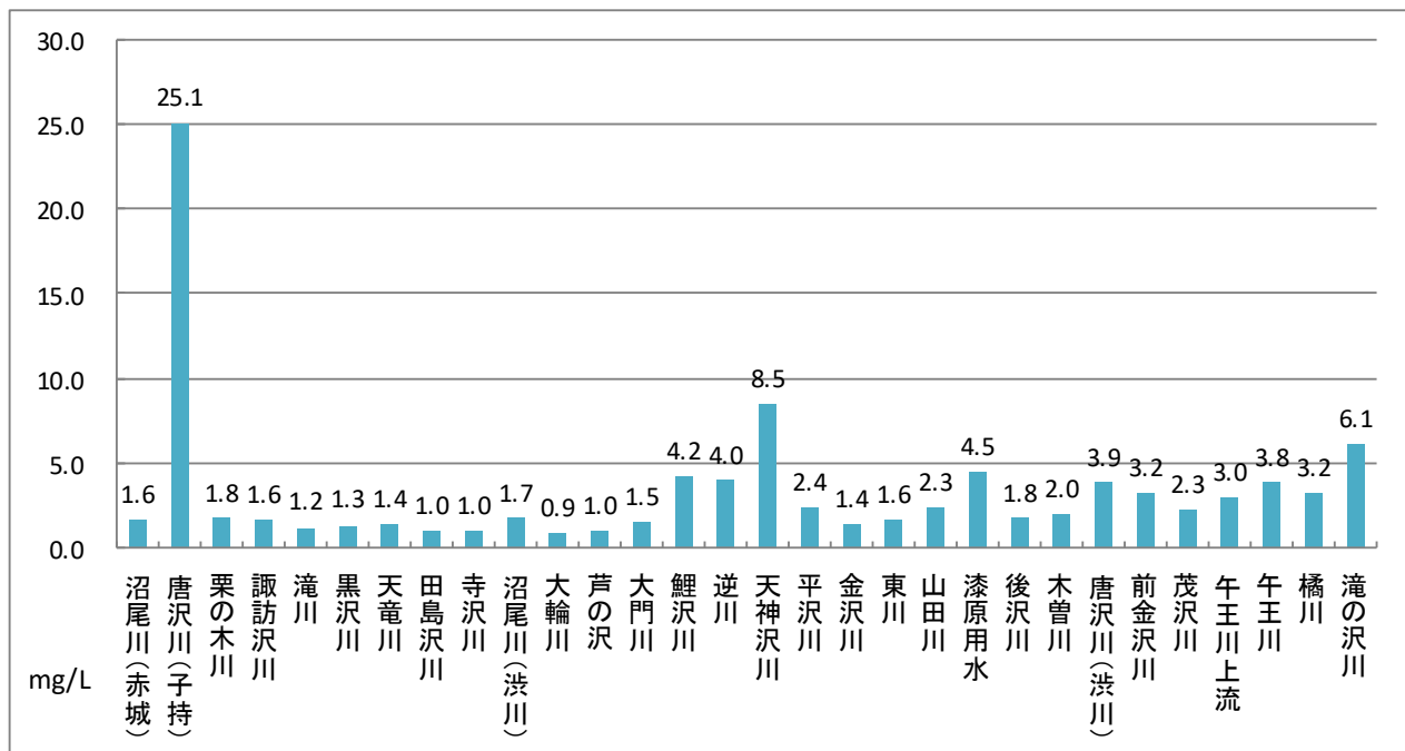
図 3－18 平成29年度中小河川のBOD年平均値
