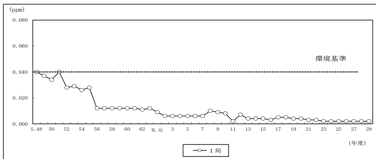
図3-2 二酸化硫黄の経年変化（日平均値の2%除外値）
