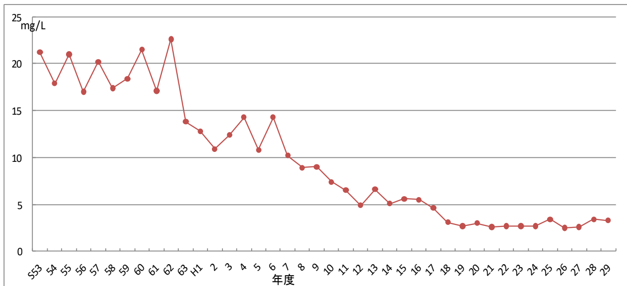
図 3－19 中小河川のBOD平均値経年変化
