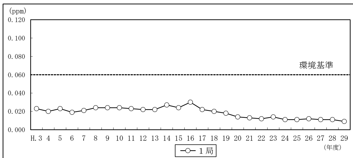
図3-3 二酸化窒素の経年変化(日平均値の98%値)
