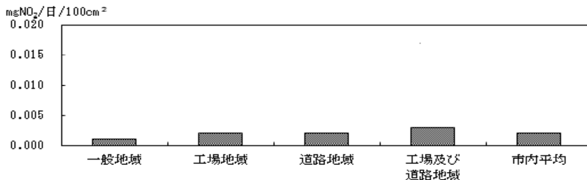
図3-9 平成29年度窒素酸化物地域別年平均値
