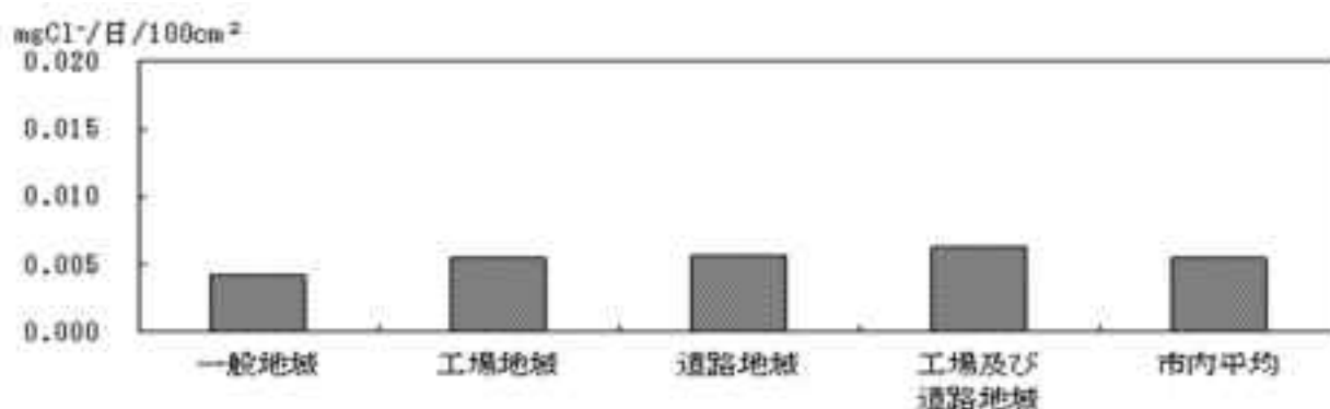
図 3-11 平成29年度塩素イオン地域別年平均値
