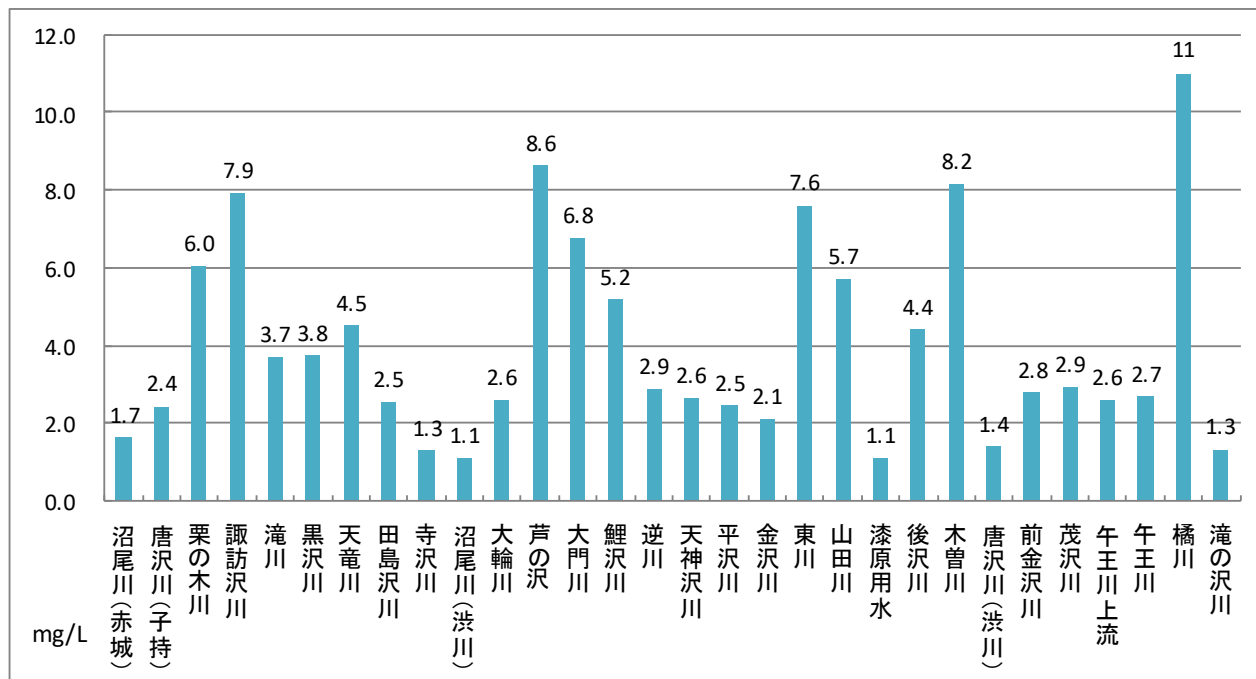
図3-17 平成29年度硝酸性窒素及び亜硝酸性窒素年平均値
