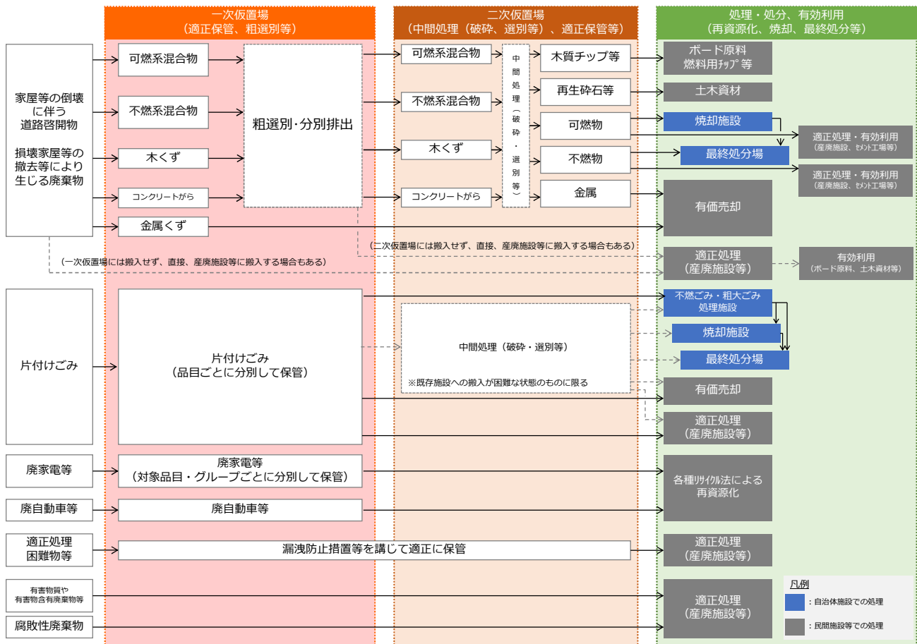
図表6-14-1 災害廃棄物の処理フロー（二次仮置場を設置する場合）
