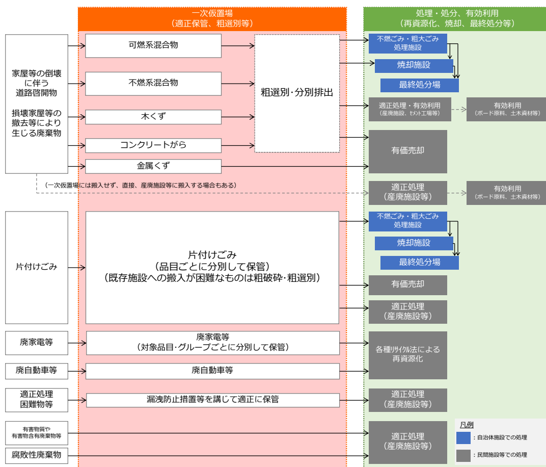
図表6-14-2 災害廃棄物の処理フロー（二次仮置場を設置しない場合）
