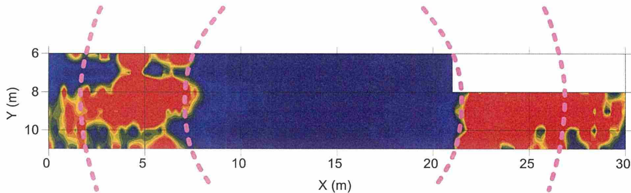
金井東裏 4 号墳 タイムスライス
