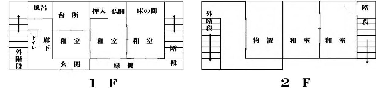
間取図
