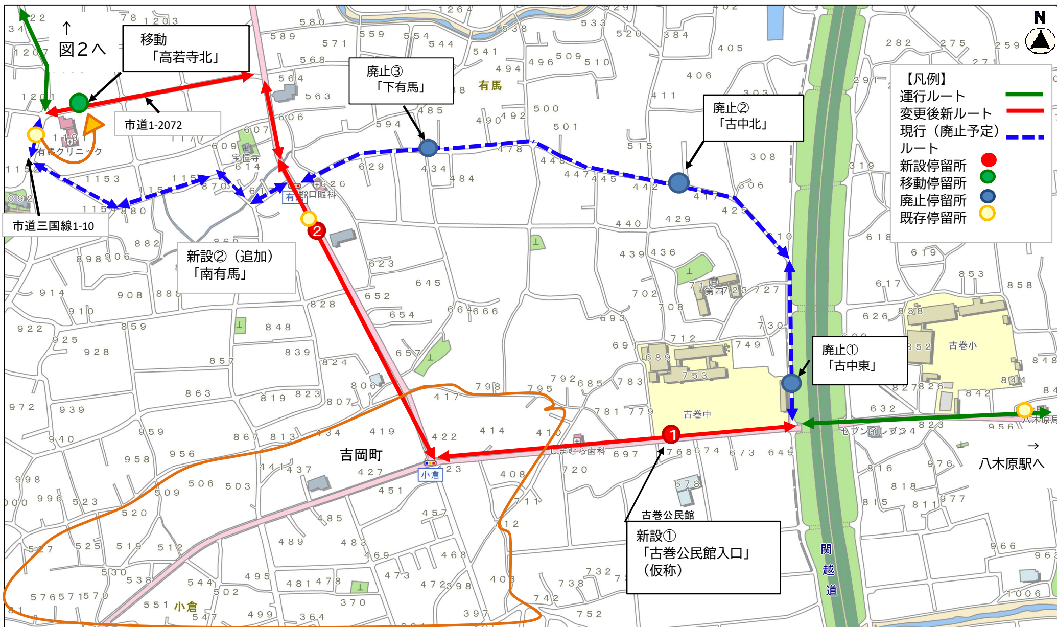
図1 渋川温泉～渋川スカイランドパーク線「古巻公民館入口」～「高若寺北」間 停留所(バス停)新設及びルート変更(案)
