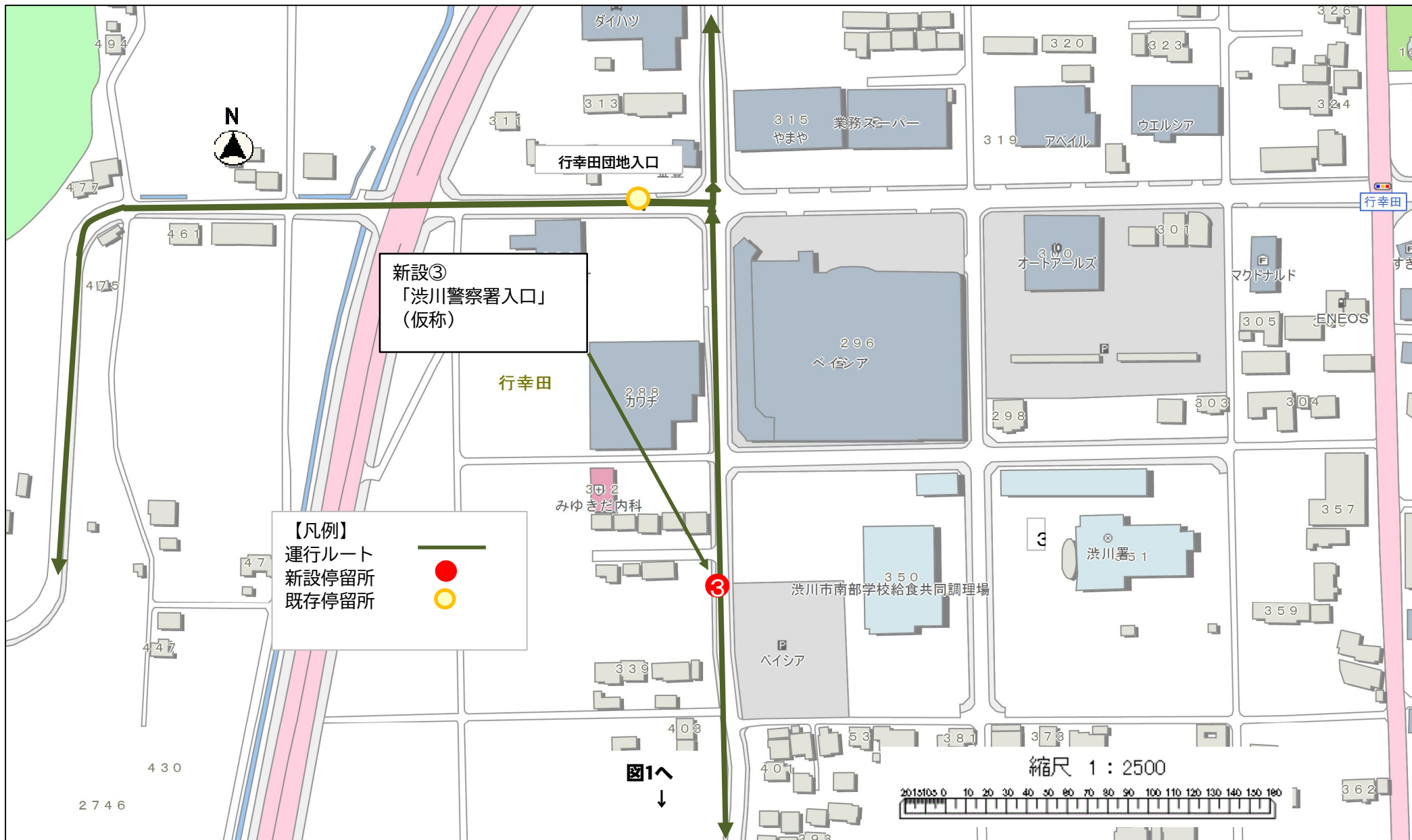
図2 渋川温泉～渋川スカイランドパーク線「渋川警察署入口」停留所(バス停)新設(案)
