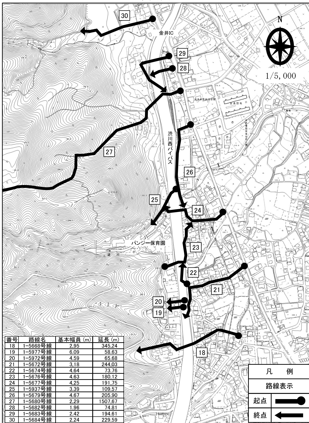
平面図2
